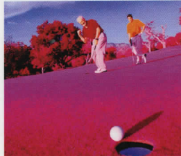
efeitos ópticos
